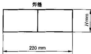
图2 格室片焊接处抗拉强度试样的示意图
